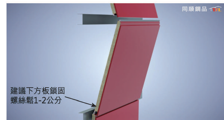
4. 插入欲更換之牆面板
