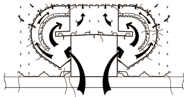
通風器擋水及排水過程示意圖
