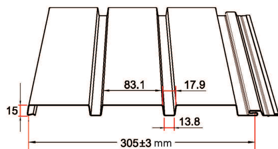
斷面圖 305P 企口板
