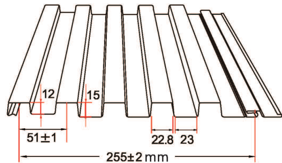
斷面圖 255K 企口板
