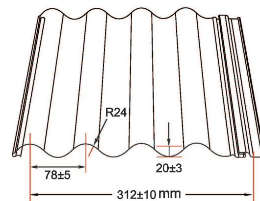
斷面圖 312 企口板
