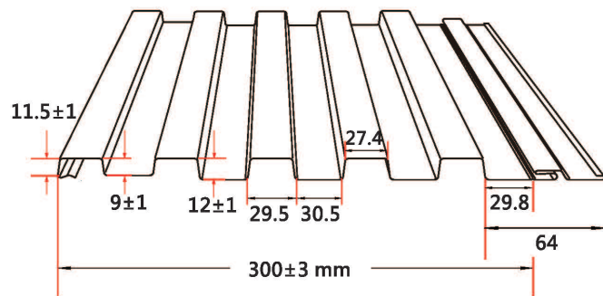
斷面圖 300K 企口板
