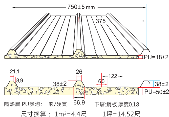
斷面圖 750 三溝PU發泡 屋頂板
