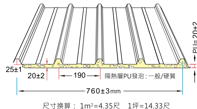
斷面圖 760型 五溝雙層發泡鋼板
