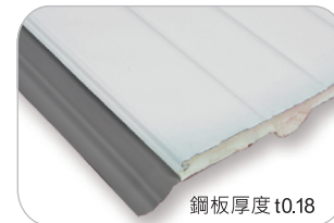
斷面圖 750 三溝PU發泡 屋頂板
