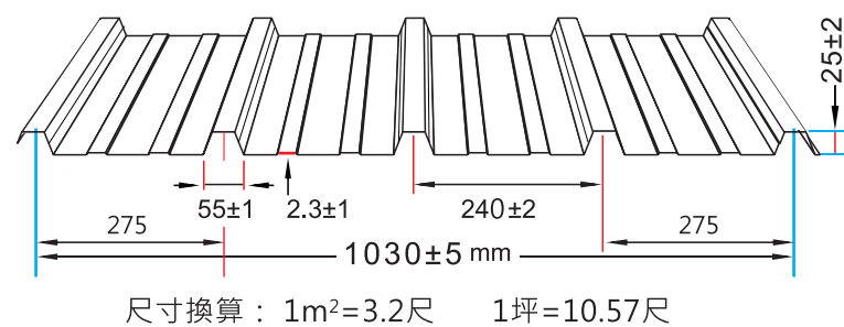
斷面圖 1030型 五溝清板(特殊4尺料鋼卷)
