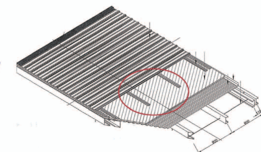
M型固定件擺放示意圖
