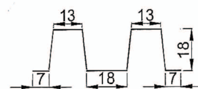
M 型固定座件 厚度:0.286(含烤漆) 短向@900mm
